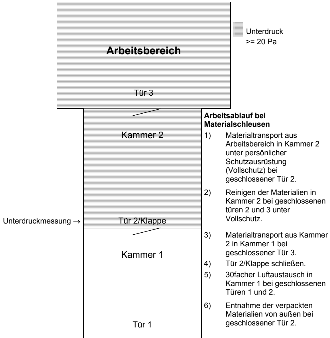
Abb. 2 Materialschleuse (Prinzipskizze)
